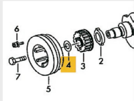
Fig. 2 Poziție instalată
